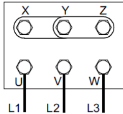
Forme d'étoile (prédéterminée) Pour tension 400V
