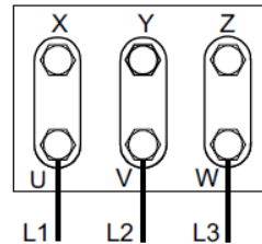
Forme triangulaire Pour tension 230V
